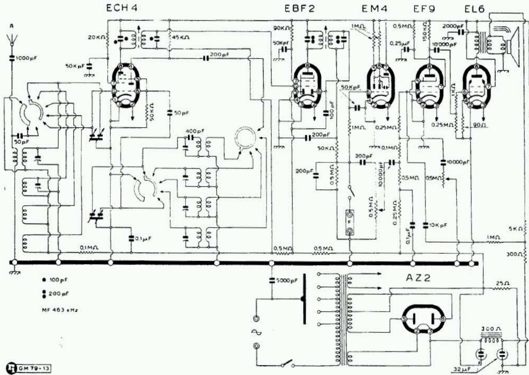
ITAL RADIO - Mod. Kosmophon «K558»
